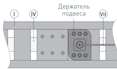
Рис. 6. Установка держателя подвеса VII на профиль I . Вид сверху
